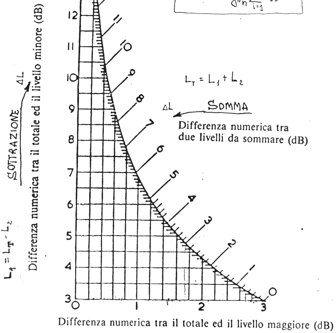
Fig. 14 - Nomogramma per sommare o sottrarre decibel.
